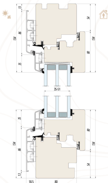
NATURO 80 ALU SYSTEEM GEMINI CLASSIC interne afsnijding onder het raamkozijn
