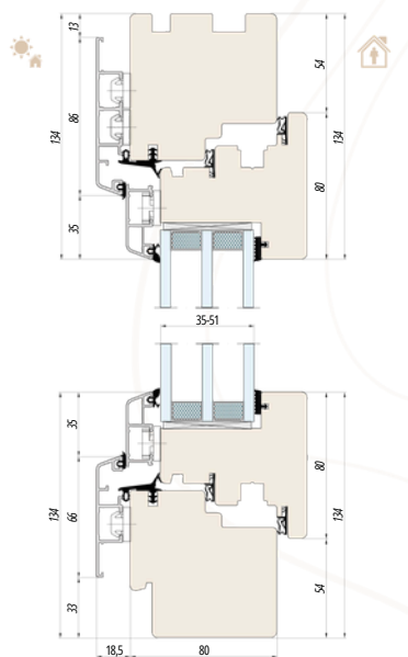
NATURO 80 ALU SYSTEEM GEMINI CLASSIC externe afsnijding onder het raamkozijn
