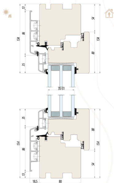
NATURO 80 ALU SYSTEEM GEMINI CLASSIC geen afsnijding onder het raamkozijn
