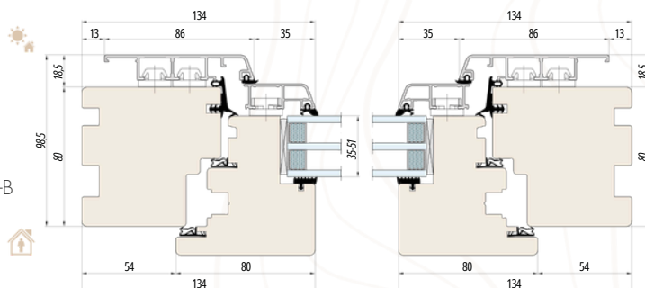
NATURO 80 ALU SYSTEEM GEMINI CLASSIC externe afsnijding onder het raamkozijn
