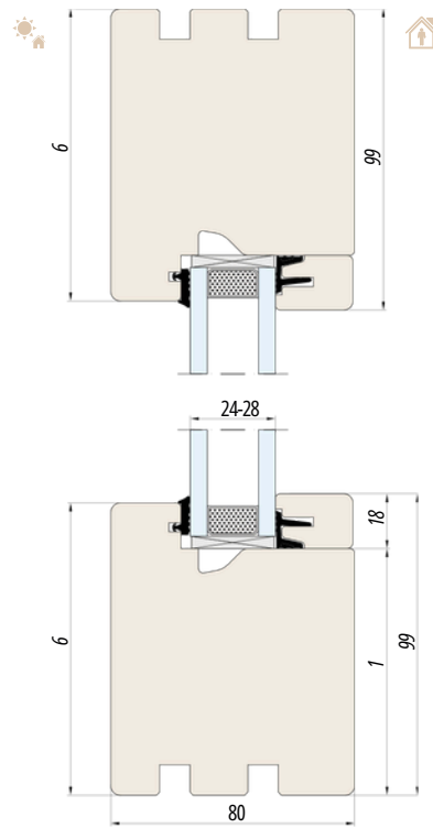
ESPERIA LIFE 80-FIX SYSTEEM geen afsnijding onder het raamkozijn
