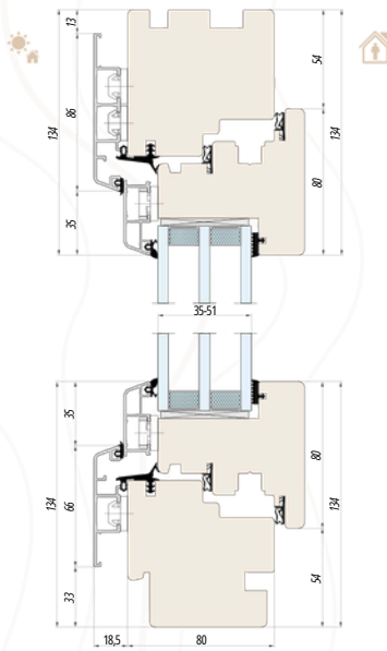
NATURO 80 ALU SYSTEEM GEMINI CLASSIC interne en externe afsnijding onder het raamkozijn
