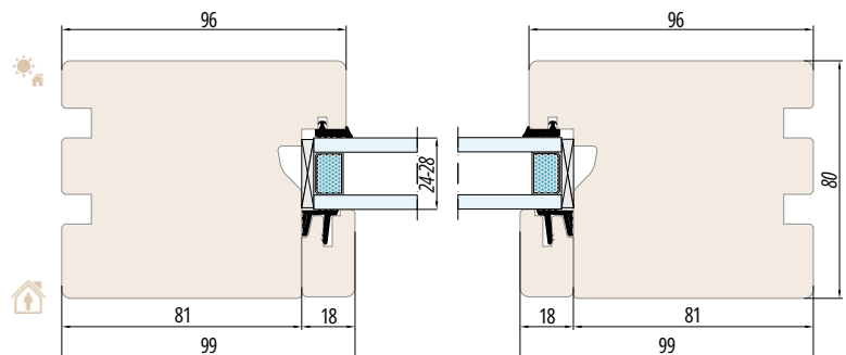
ESPERIA LIFE 80-FIX SYSTEEM HORIZONTAAL DOORSNEDE B-B
