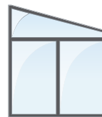
trapezium
